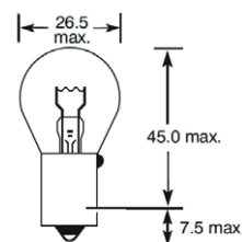
BA15s
