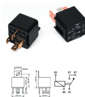
6010004 Relé spínací 12V 30A, 4 kontakty, s úchytem
