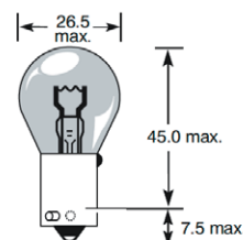
BAU15s
